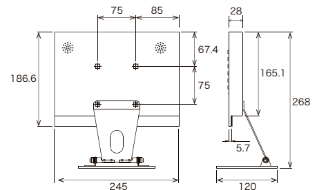
製品寸法(単位:mm)
