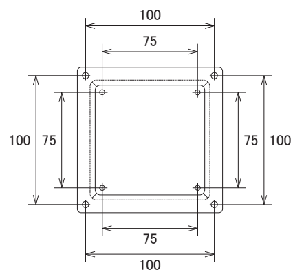
VESA100対応付属品
