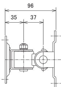
上面図
