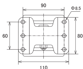
壁面取付部分前面図
